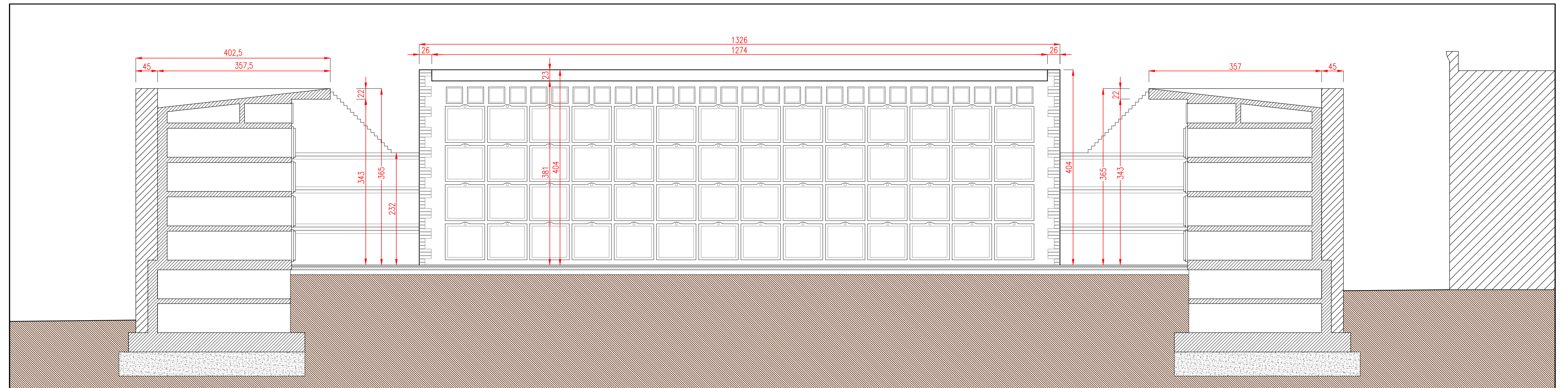
SEZIONE A'-A'
